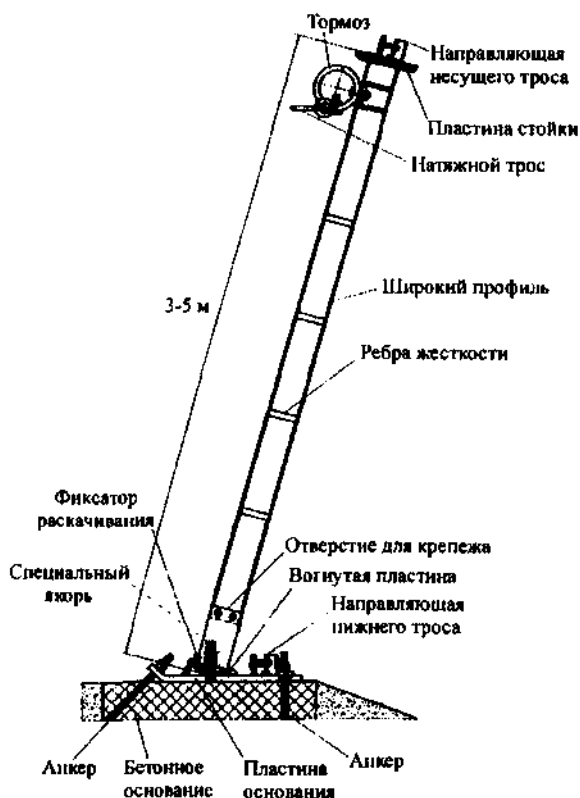
Рис. 34. Стойка барьера
