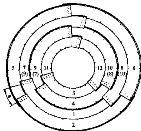
Рис. 19. Монтажная схема МГТ отверстием 1,5 м (вид с торца): а — величина сдвижки продольных стыков; цифрами показан порядок установки элементов при сборке МГТ
