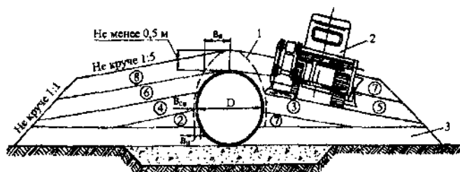
Рис. 25. Технологическая последовательность и схема послойного уплотнения грунта засыпки МГТ виброударной машиной для стесненных условий:
