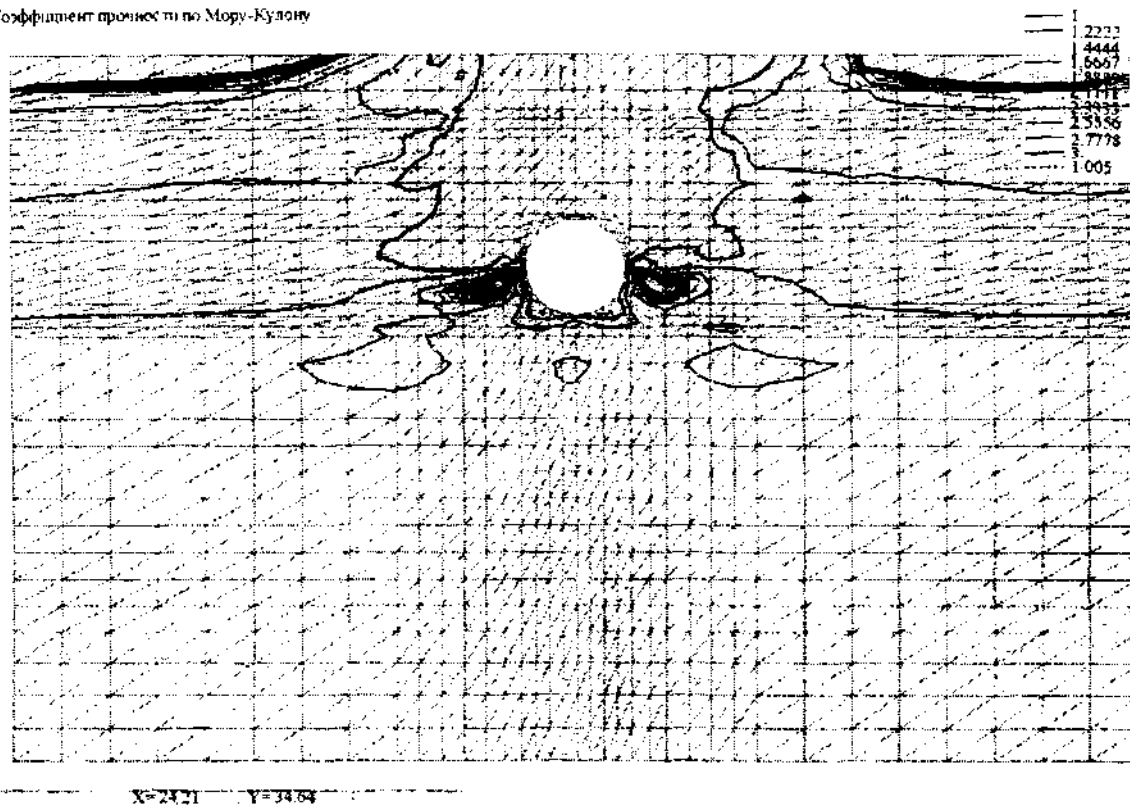
Рис. В.7. Коэффициент прочности по Морю-Кулону
