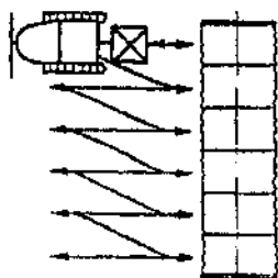
Рис. 24. Схема уплотнения грунта виброударной машиной челночным способом
