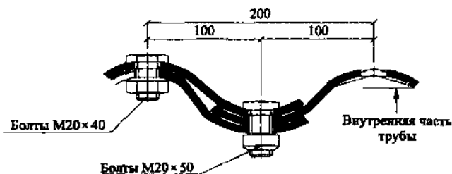
Рис. Б.3. Перекрывание листов
