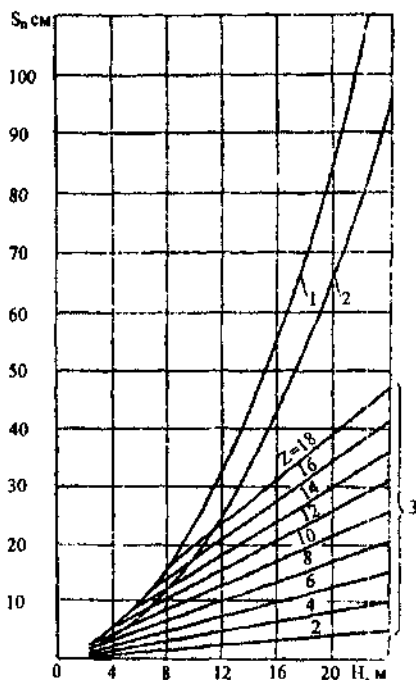
Рис. Г.1. Расчетный график для определения осадок МГТ: S_n — осадка основания при модуле деформации грунта 100 \text{ кгс/см}^2 ; H — высота насыпи; Z — расстояние от нижней границы рассматриваемого слоя до поверхности основания; 1 — при однородном основании и \gamma = 1 \text{ т/м}^3 ; 2 — то же, при \gamma = 1,7 \text{ т/м}^3 ; 3 — при неоднородном основании и Z = 2-18 \text{ м}
