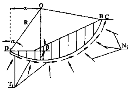
Рис. Ж.2. Принципиальная схема метода КЦПС
