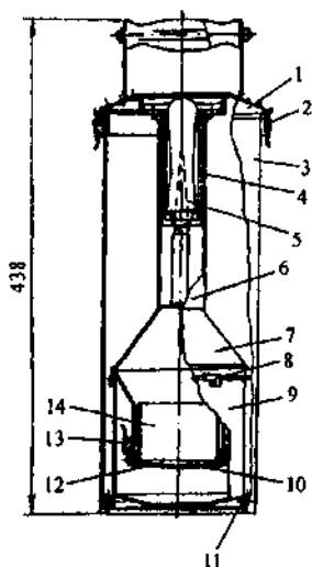
Рис. Л.1. Схема плотномер-влажмера Н. П. Ковалева: 1 – верхняя крышка; 2 – замок; 3 – футляр; 4 – насадка; 5 – нож; 6 – трубка; 7 – поплавок; 8 – крючки; 9 – сосуд; 10 – тарировочный груз; 11 – резиновое кольцо; 12 – нижняя крышка; 13 – замок; 14 – режущий цилиндр
