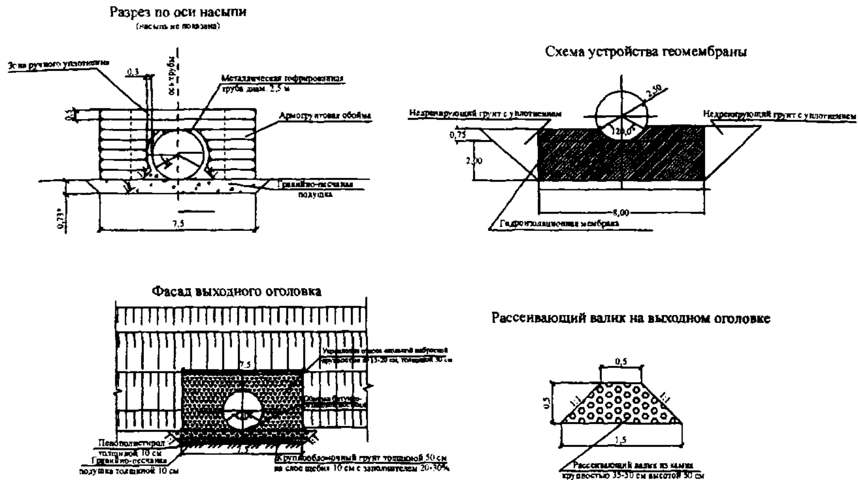
Рис. М.2. Пример проектирования армогрунтовой обоймы, противофильтрационного экрана (геомембраны), входного и выходного оголовка и рассеивающего валика для МГТ на рис. М.1
