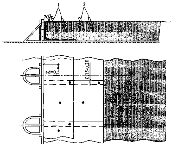
Рис. 32. Укладывание с натяжением на уплотненную поверхность грунта выпущенных за внешнюю грань щитов армирующих полотнищ и закрепление их колышками:
