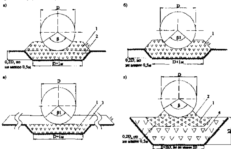
Рис. 7. Конструкция основания:
