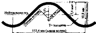
Рис. А.2. Профиль гофрированного листа Толщина листа 3,0-7 мм, углы изгиба гофра 44,53-46,08°, Прямая оставка 43,24-47,88 мм
