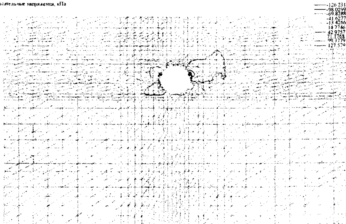
Рис. В.6. Касательные напряжения
